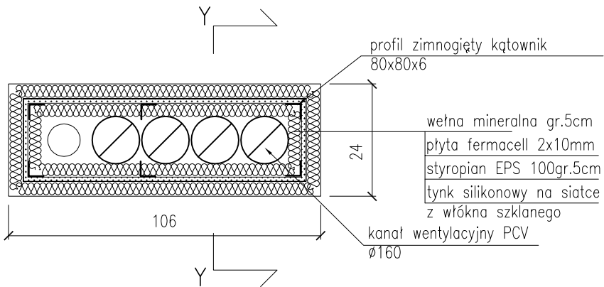
PRZEKRÓJ PRZEZ KOMIN – ponad połacią
