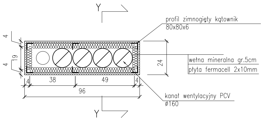
PRZEKRÓJ PRZEZ KOMIN – na strychu
