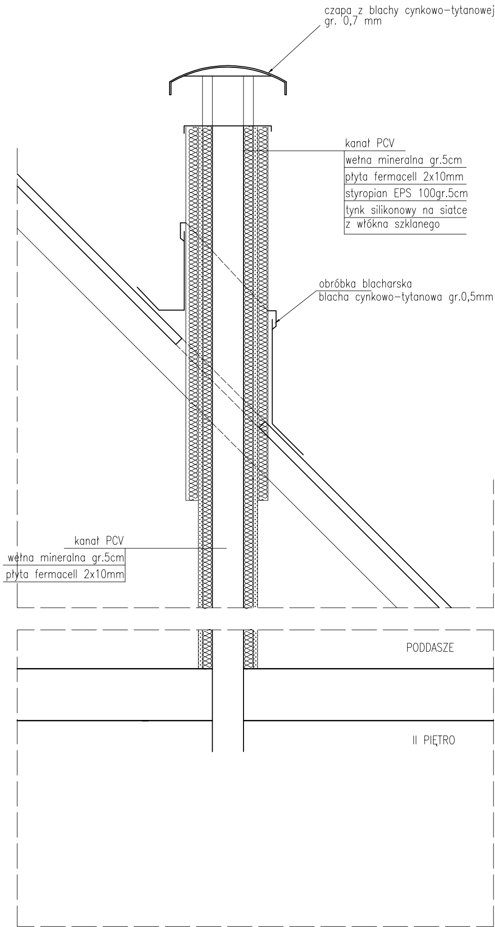
PRZEKRÓJ PRZEZ KOMIN Y–Y
