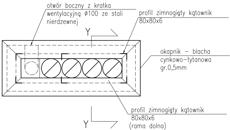
SZCZEGÓŁ ZAKOŃCZENIA KANAŁÓW
