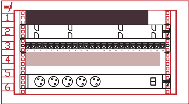
Punkt Dystrybucyjny PD 1/1 szafa rack 600x400 6U
