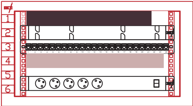
Punkt Dystrybucyjny PD 0/1 szafa rack 600x400 6U
