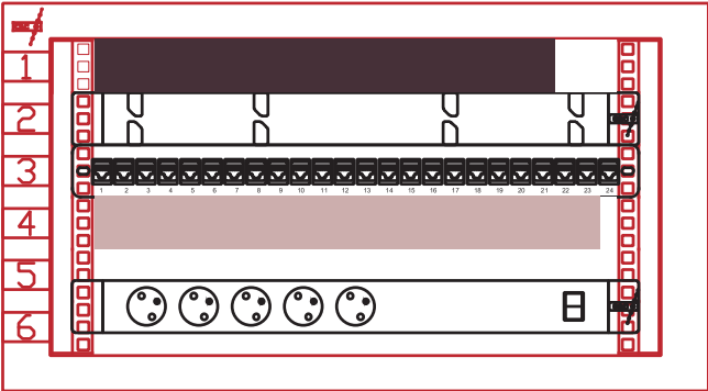
Punkt Dystrybucyjny PD 1/2 szafa rack 600x400 6U
