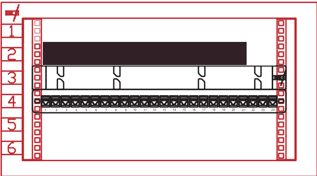
Punkt Dystrybucyjny PD P/1 szafa rack 600x400 6U
