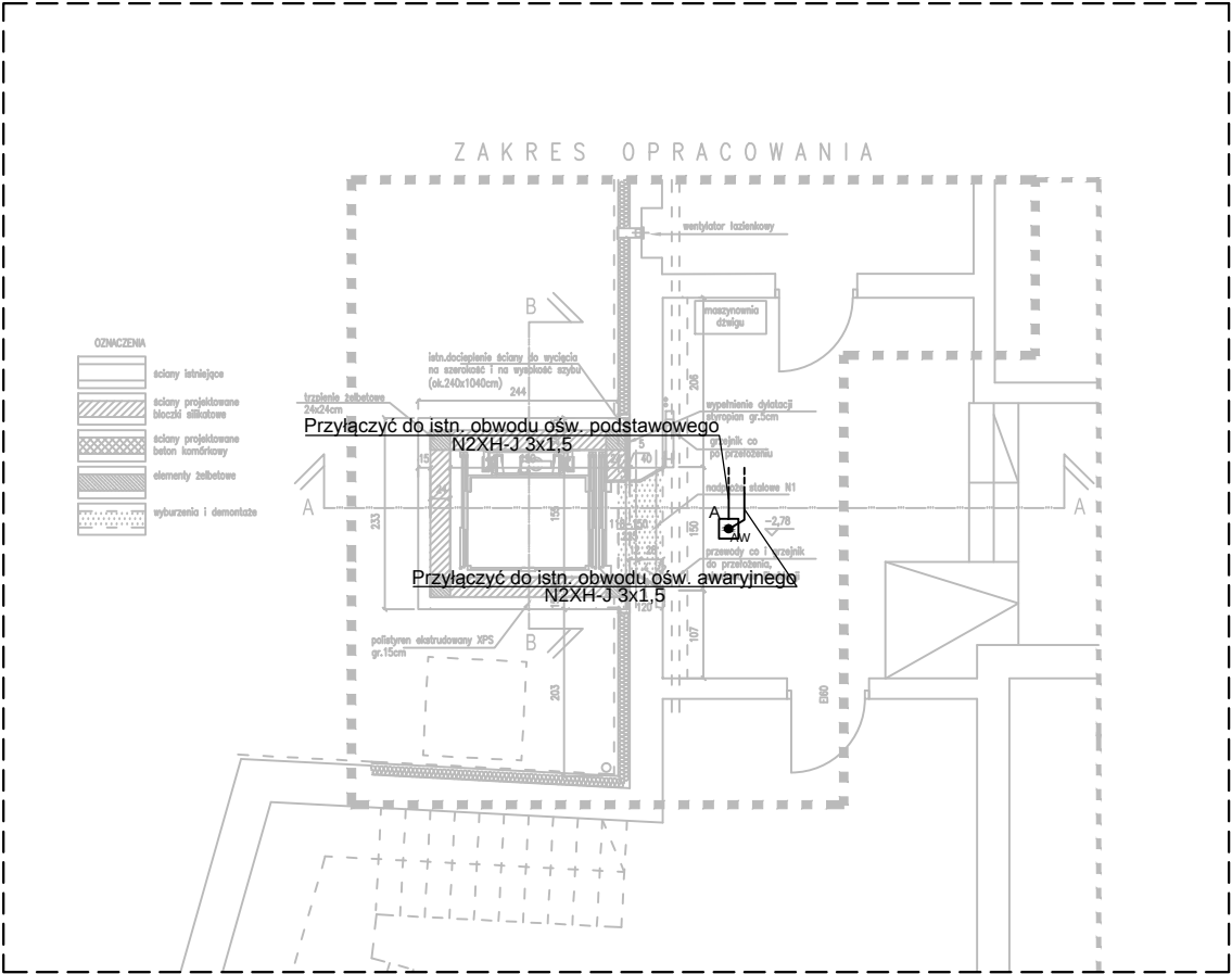
Rzut piwnicy
