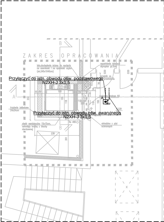
Rzut I piętra
