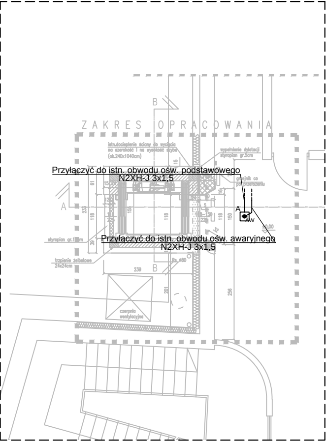
Rzut parteru
