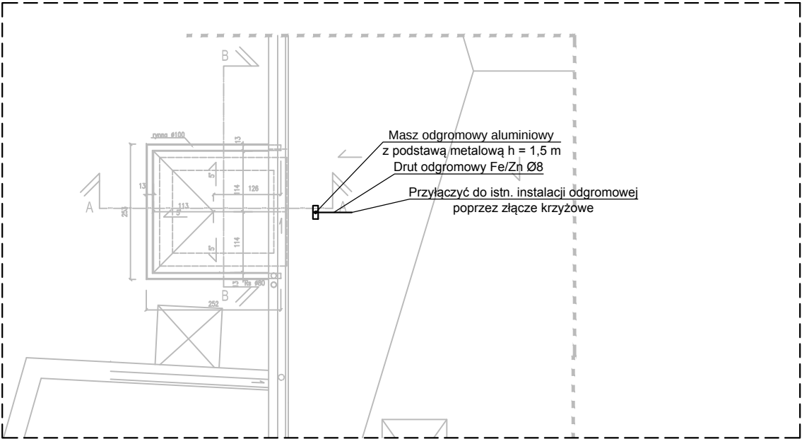
Rzut dachu
