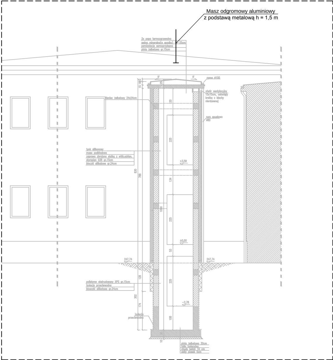
Przekrój B
