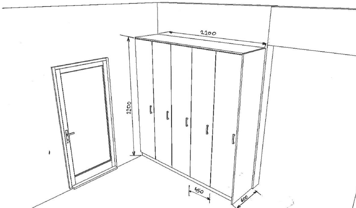
Rys. 3 Szafa pięciodrzwiowa
