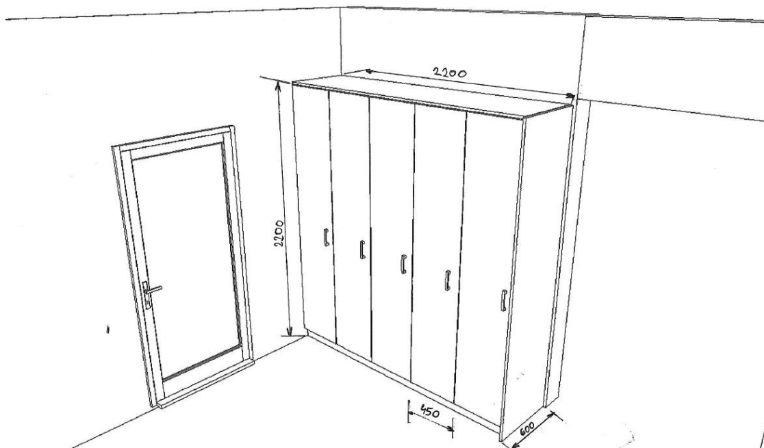
Rys. 3 Szafa pięciodrzwiowa
