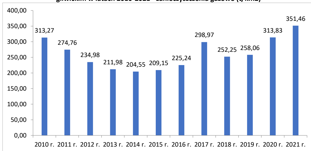
Wykres 1. Emisja zanieczyszczeń powietrza z zakładów szczególnie uciążliwych w powiecie gliwickim w latach 2010-2021 - zanieczyszczenia gazowe (t/km 2 )
