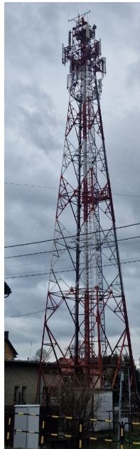
Widok obiektu wraz z zainstalowanym zespołem antenowym
